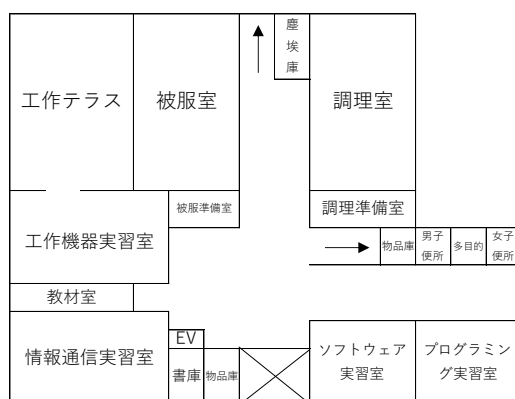
キタミライ棟・1階平面図（→は階段を表す）
