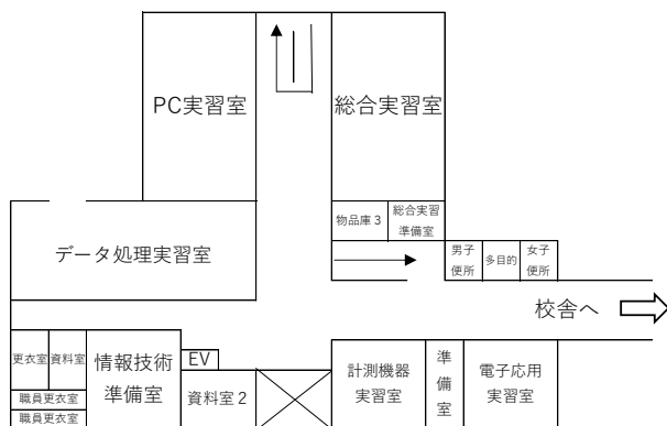
キタミライ棟・2階平面図（→は階段を表す）
